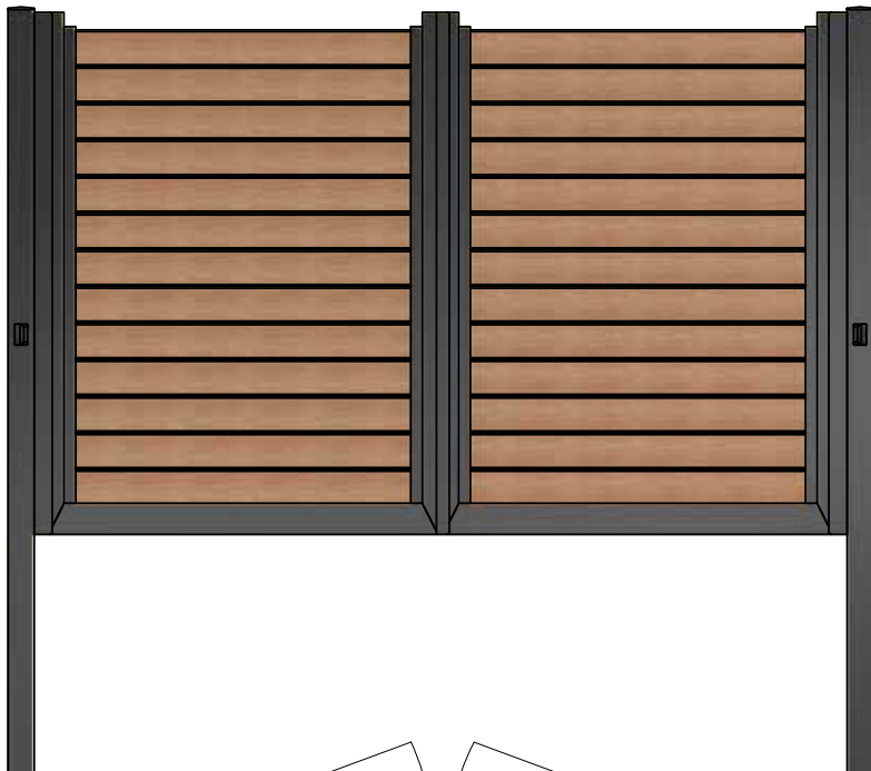
Frontansicht Tor
