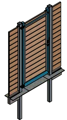
Rückansicht Tür
